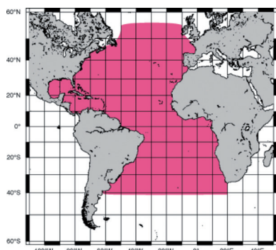
大西洋におけるメバチの分布
