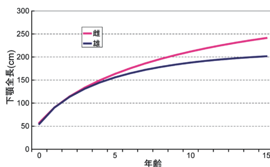
図 5. 雌雄別の成長曲線（Sun et al. 2002）
