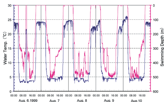
図 3. アーカイバルタグから得られた親潮前線域でのメカジキの日周鉛直移動データ 移動データは 1999 年 8 月 6～10 日のもの。赤線が水深、水色線が水温を示す。
