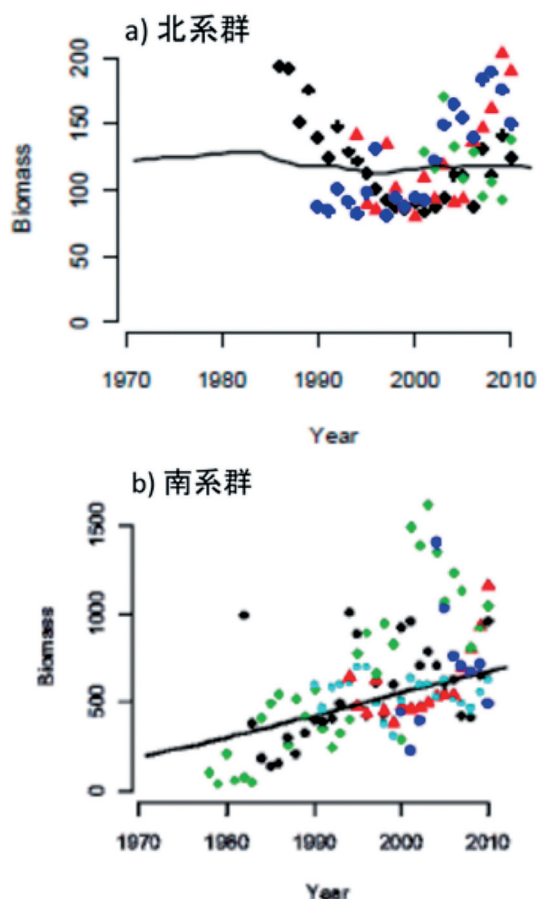
図 6. 大西洋のアオザメにおいて BSP によって推定されたバイオマス（黒実線）と各国の提出した CPUE（マーカー）のトレンド（a：北系群、b：南系群）（ICCAT 2012） CPUE を示すマーカーは、北大西洋では黒が米国、赤が日本、緑がポルトガル、青がスペイン、南大西洋では黒がウルグアイ、緑がブラジル、青がポルトガル、水色がスペインを示す。いずれも 1971 年を開始年とし、CPUE に国別の重み付けをしていない。
