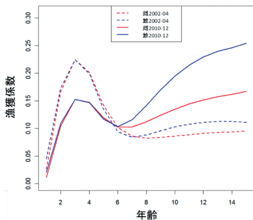
図 6. 北太平洋ビンナガ資源への雌雄別、年齢別の漁獲係数の近年(2010～2012 年平均)と 2002～2004 年平均との比較
