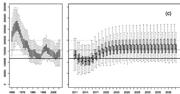
図 8. 北太平洋ビンナガ資源の将来予測（上図：加入レベル平均（1966～2012 年）、中図：加入量低位、下図：加入量高位） 各パネルの縦軸は産卵資源量。各パネルの左のパネルは過去（1966～2011 年）。右のパネルが将来予測で、白いバーは F が 2010～2012 年の平均の場合。灰色のバーは F が 2002～2004 年の平均の場合。また、横に伸びる破線、灰色実線、破線及び黒い実線は上から 75 パーセンタイル、中央値、25 パーセンタイル、過去最小から 10 番目までの SSB（産卵資源量）の平均。
