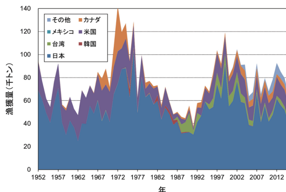
図 1. 北太平洋ビンナガの漁法別漁獲量（上図）、国別漁獲量（下図）
