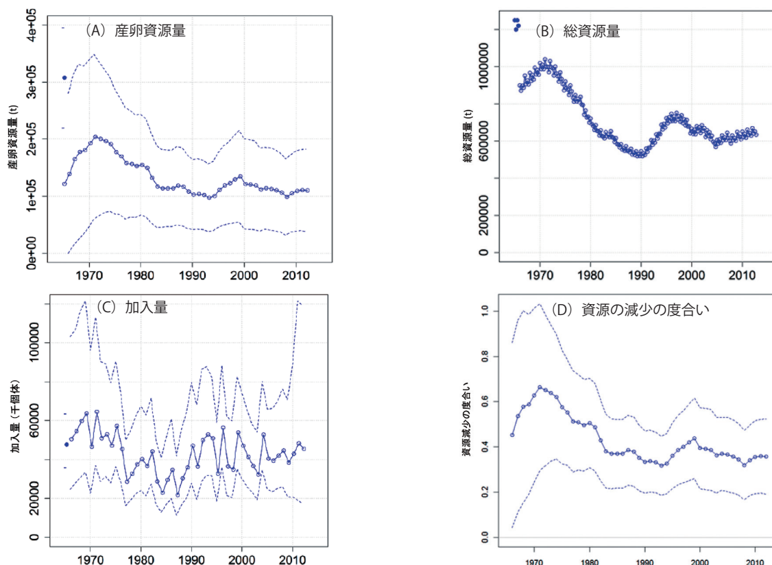
図 5. 北太平洋ビンナガの (A) 産卵資源量、(B) 総資源量、(C) 加入量、(D) 資源の減少の度合い ( SSB/SSB_0 ) (ISC 2014) 点線はその推定値の 95% 信頼区間。総資源量は四半期単位、それ以外は年単位で示されている。
