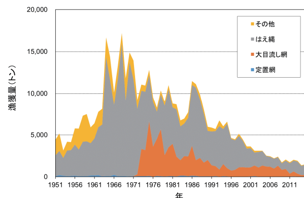
図 1. 北太平洋（赤道以北）におけるマカジキの我が国の漁業種別漁獲量（ISC 2016）
