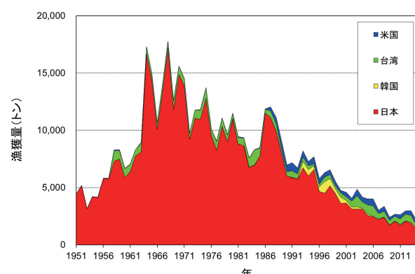
図 2. 北太平洋におけるマカジキの国別漁獲量（ISC 集計分）（ISC 2016）
