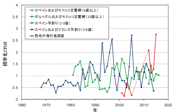
図 4. 大西洋クロマグロ（東系群）の資源評価に用いた CPUE（ICCAT 2017a）
