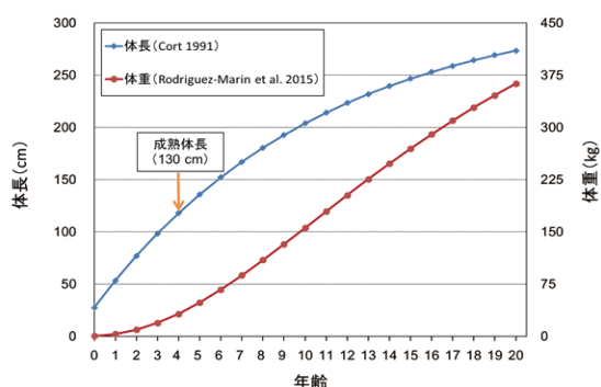
図2. 大西洋クロマグロ(東系群)の年齢あたりの体長(青線)と体重(赤線)(ICCAT 2017b) 図中の矢印は成熟体長を表す。
