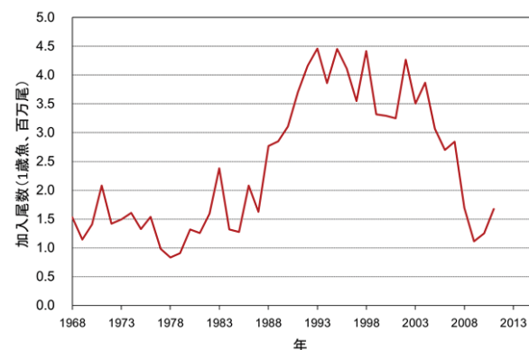
図 6. 大西洋クロマグロ（東系群）の加入尾数（1 歳魚）の経年変化 資源評価モデルで推定した加入尾数（ICCAT 2017a）。
