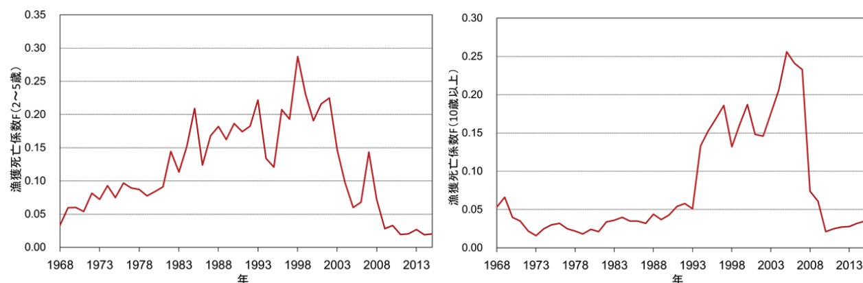
図 7. 大西洋クロマグロ（東系群）の 2～5 歳（左図）及び 10 歳以上（右図）の漁獲死亡率係数 F（ICCAT 2017a）
