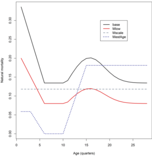
図 15. 第 18 回熱帯まぐろ作業部会（2016 年）に資源評価で使用された年齢別自然死亡率（M）（黒実線）（X 軸は四半期スケール）（Langley 2015） Base は資源評価ベースモデル用、Mlow は SS3 感度解析に用いられた低い値。
