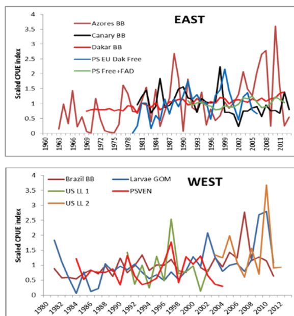
図 6. 東部大西洋 (上) 及び西部大西洋 (下) におけるカツオ CPUE の経年変化 (ICCAT 2017)
