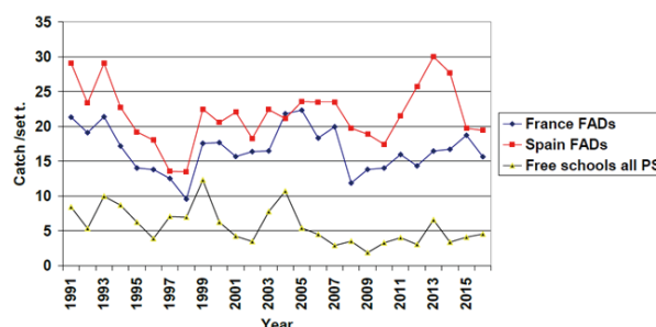
図 3. 東部大西洋におけるまき網によるカツオ漁獲率 (1 操業あたり漁獲量) の経年変化 (ICCAT 2017)
