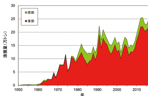
図 1. 東部及び西部大西洋におけるカツオ漁獲量の年変化 (ICCAT 2017 を改変)
