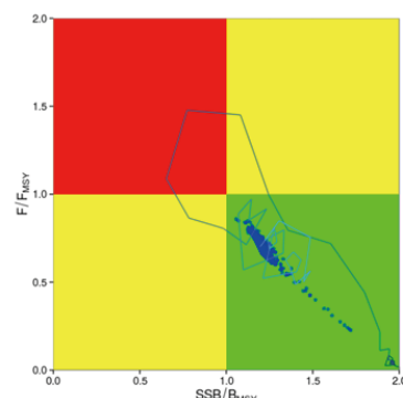
図 7. Schaefer 型の ASPIC から推定された西部大西洋のカツオにおける B/B_{MSY} と F/F_{MSY} の歴史的推移 (ICCAT 2017)
