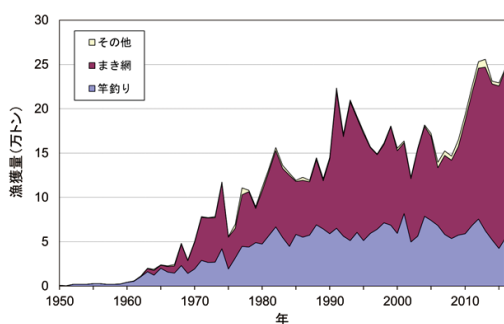
図 2. 大西洋におけるカツオの漁法別漁獲量の年変化 (ICCAT 2017 を改変)
