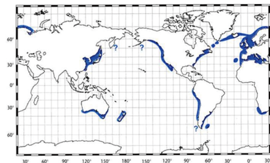
図 1. ウバザメの分布 (Last and Stevens 1994、内田 1995)
