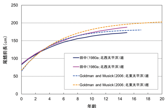
図 4. ネズミザメの年齢と成長 (田中 1980a, Goldman and Musick 2006)
