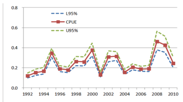
図 7. ミナミマグロ漁場において、日本の科学オブザーバーが収集したデータを基に標準化したニシネズミザメの CPUE (松永ほか 2012)
