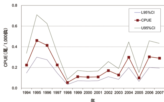
図 6. 北太平洋における日本のえ縄漁業データを基に標準化したネズミザメの CPUE
