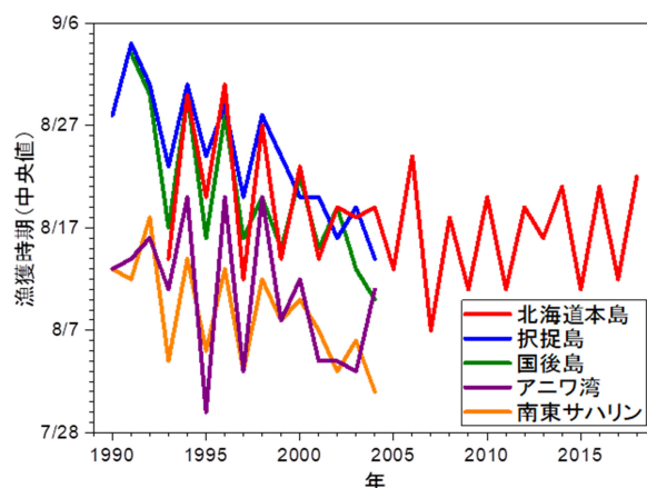
図 8. 北海道本島および周辺地域のカラフトマスの漁獲時期の経年変化 (北海道本島以外のデータは、Kaev et al. 2007、Kaev and Romasenko 2007 から引用)
