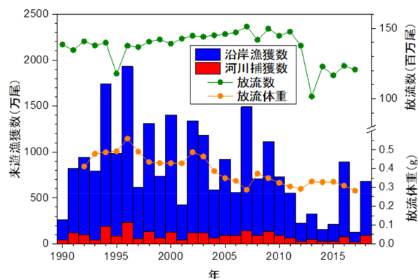
図 6. 日本系カラフトマスの來遊漁獲数、放流数および放流体重の推移 (歴史的データは付表 1 参照)
