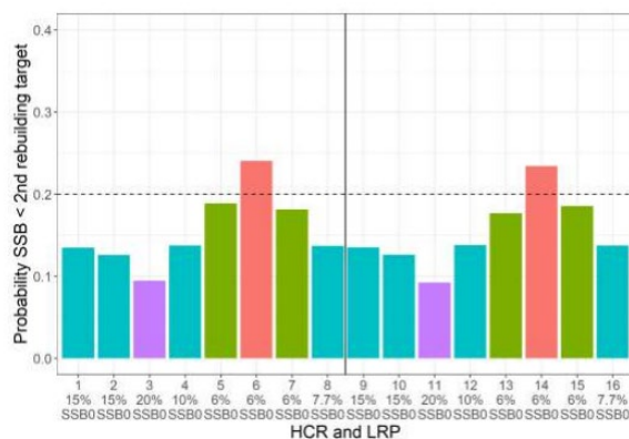
図 5.管理戦略候補を評価するための MSE のアウトプットの一例（ISC 2025）
