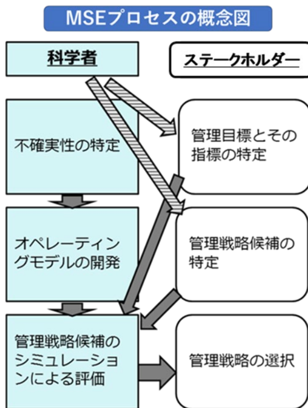
図3. MSE の進め方に関する概念図 色の付いたボックスは主に科学者が策定し、白いボックスは主にステークホルダー (行政官を含む) が策定する (Punt et al. 2016)。 斜線の矢印はアドバイスを示す。
