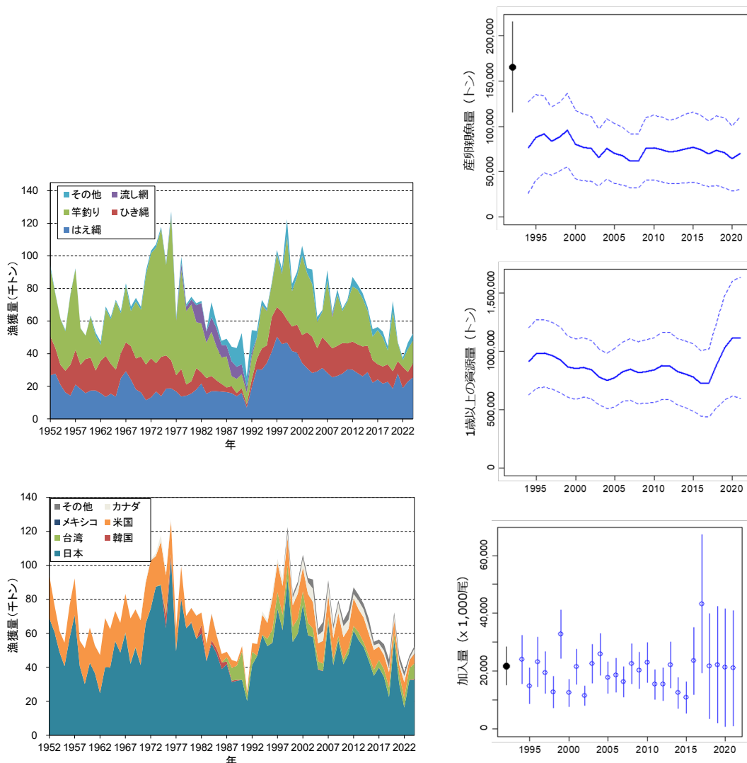
北太平洋ビンナガの雌の産卵資源量 (上)、 1歳以上の資源量 (中央)、加入量 (下) 上2図の実線及び下図の○印はいずれも推定値の中央値。 上2図の破線及び下図の縦棒は推定値の95%信頼区間。左 端の●印及び縦線 (黒) は、それぞれ平衡状態における漁獲 がない場合の雌の産卵親魚量及び加入量を示す。
