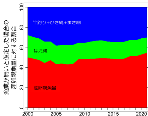
図6. 北太平洋ビンナガ資源への各漁業のインパクト(2000~2021年) 縦軸は、漁業が無かったと仮定した場合の産卵資源量を100とした時の各漁業のインパクトの割合を示す。 青色: 釣り+ひき縄+まき網、緑: はえ縄、赤: 産卵資源量
