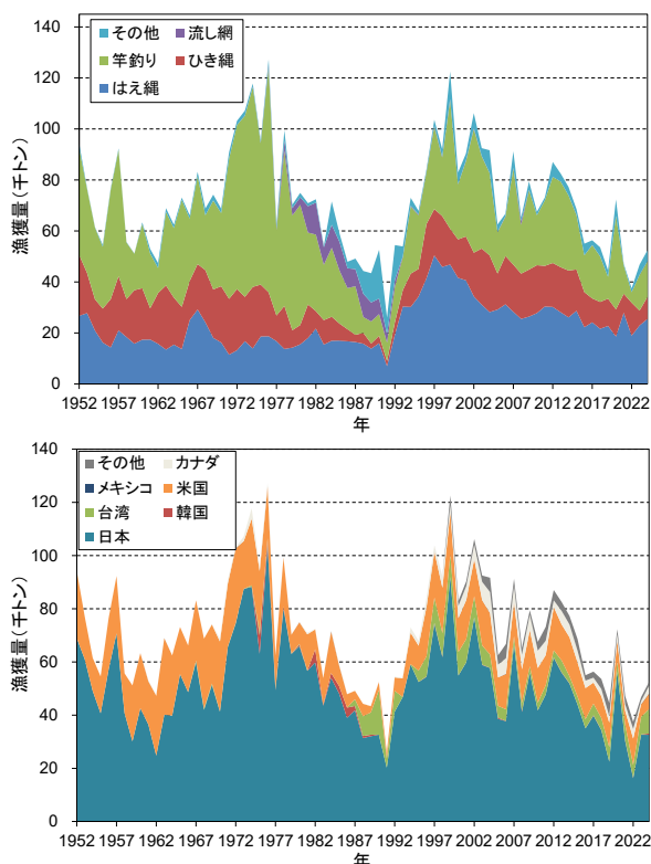
図1. 北太平洋ビンナガの漁獲量の変遷 (1952～2024年) (上図) 漁法別漁獲量、(下図) 国・地域別漁獲量 (ISC 2025、WCPFC 2025) なお、2024年の漁獲量は暫定値。
