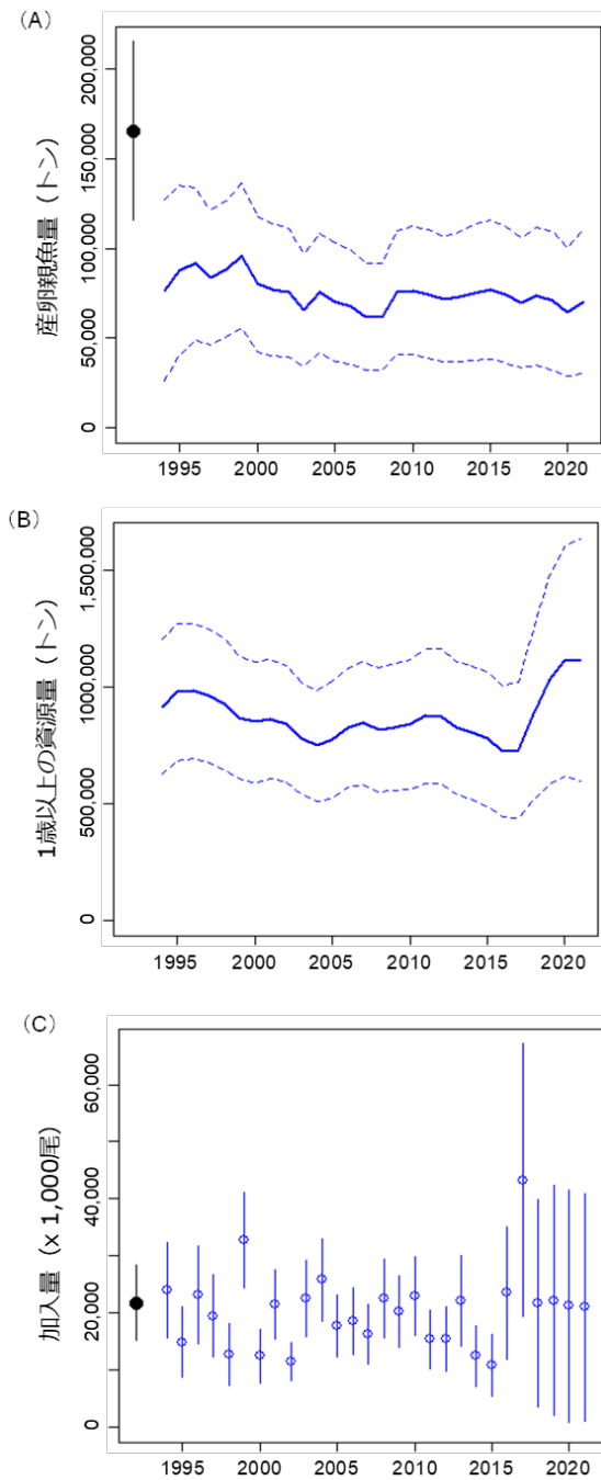
図4. 北太平洋ビンナガの (A) 雌の産卵親魚量、(B) 1歳以上の資源量、(C) 加入量推定値(1994~2021年、ISC 2023) (A)、(B)の実線及び破線はそれぞれ推定値の中央値及び95%信頼区間、(C)の○印及び縦棒はそれぞれ推定値の中央値及び95%信頼区間。 (A)、(C)の左端の●印及び縦線(黒)は、それぞれ平衡状態における漁獲がない場合の雌の産卵親魚量及び加入量を示す。
