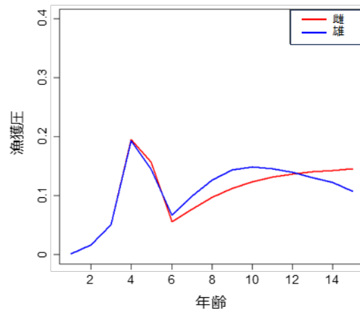
図5. 北太平洋ビンナガ資源への雌雄別、年齢別の漁獲率(赤:雌、青:雄)
