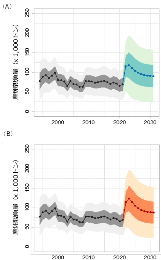
図7. 北太平洋ビンナガ資源の将来予測結果 (将来予測期間は2022~2031年) (A) : 漁獲圧一定 ( F_{2018-2020} ) シナリオでの雌の産卵親魚量 (B) : 歴史的な漁獲圧 ( F_{2005-2019} ) を用いたシナリオでの雌の産卵親魚量 それぞれの実線は平均値、濃淡の範囲は60%と95%の信頼区間を示す。
