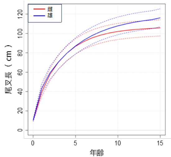
図3. 北太平洋ビンナガの雌雄別の成長曲線 (ISC 2023) 点線は95%信頼区間。
