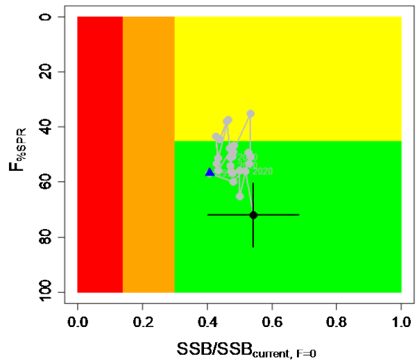
図8. 資源評価期間(1994~2021年)の漁獲圧( F_{\%SPR} )と限界管理基準値( 14\%SSB_{current, F=0} )及び閾管理基準値( 30\%SSB_{current, F=0} )に対する産卵親魚量( SSB/SSB_{current, F=0} )の推移(ISC 2023) 縦軸の F_{\%SPR} は、漁獲が無いときのSPR(Spawning Per Recruitment: 加入量当たりの産卵親魚量)に対して漁獲した残るSPRの割合を示す。 赤色区間は限界管理基準値( 14\%SSB_{current, F=0} )以下、橙色区間は限界管理基準値から閾管理基準値( 30\%SSB_{current, F=0} )まで、黄区間は F_{\%SPR} が目標管理基準値( F_{45\%SPR} )以下、緑色区間は目標管理基準値( F_{45\%SPR} )以上を示す。青三角点は資源評価期間の開始年(1994年)の推定値、黒点と縦横棒は2021年の推定値と95%信頼区間を示す。
