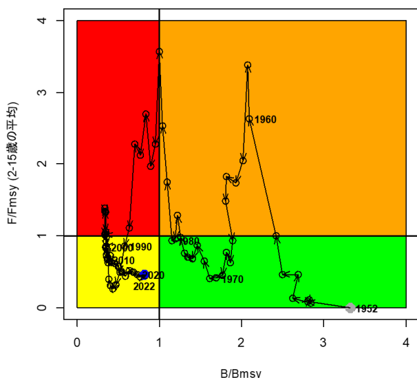
図8. ミナミマグロ資源の神戸プロット:MSYを産出する資源量に対する各年の資源量の比 ( B/B_{msy} :横軸)及びMSY水準を与える漁獲死亡率に対する各年の漁獲死亡率の比 ( F/F_{msy} :縦軸)の推移(1952~2022年) 丸印は推定されたそれぞれの比の中央値を示し、矢印はそれらの推移を示す。灰色の丸印は1952年時点、青色の丸印は2022年時点(資源の現状)。CCSBT(2023)のデータを基に作図。
