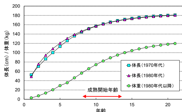
図 4. CCSBT で用いられているミナミマグロの成長曲線 体長 (尾叉長) に関しては、比較のため、1970 年代と 1980 年代生まれの年級群に対応する成長曲線のみを示した。 1970 年代以前、1980 年代以降に対応する体長の曲線はそれぞれ 1970 年代、1980 年代のものと同様のカーブを描く。 体長の曲線は Eveson (2011) の式を基に、体重の曲線は本文の式を基にそれぞれ作図。
