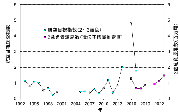
図6. 航空目視調査によるミナミマグロの加入量指数及び遺伝子標識調査による 2 歳魚資源尾数推定値 (1993~2019 年、2021~2023 年)
