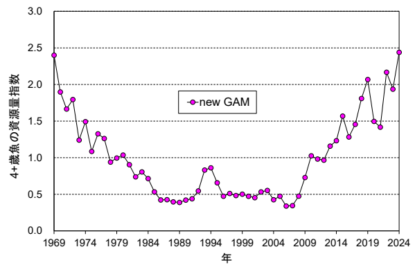
図5. 日本のはえ縄漁業の CPUE データに基づくミナミマグロの 4+歳魚の資源量指数 (1969~2024 年) Itoh and Takahashi (2025) のデータを基に作図。
