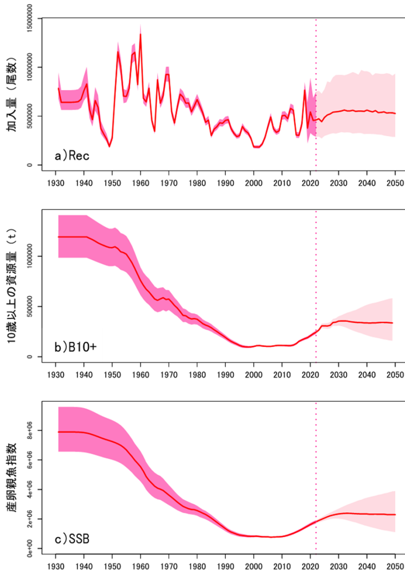
図7. 2023年に資源評価モデルにより推定されたミナミマグロの加入量 (Rec：上段)、10歳以上の親魚資源量 (B10+：中段) 及び親魚資源量 (SSB：下段) (1930～2050年) B10+は以前に用いられていた定義による親魚資源量、SSBは産卵ポテンシャルに基づく「総再生産出力 (Total Reproductive Output：TRO)」による親魚資源量を表す。太線は中央値、影部は80%確率区間を示す。縦の点線は2022年(資源の現状)を指す。2023年からの将来部分は管理方式(ケーブタウン方式)を用いてTAC設定を続けた場合の予測である。 CCSBT科学委員会が2023年に実施した資源評価の結果を基に作図 (CCSBT 2023)。
