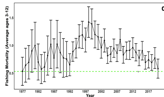
統合モデルの解析結果 (1977~2020 年)
