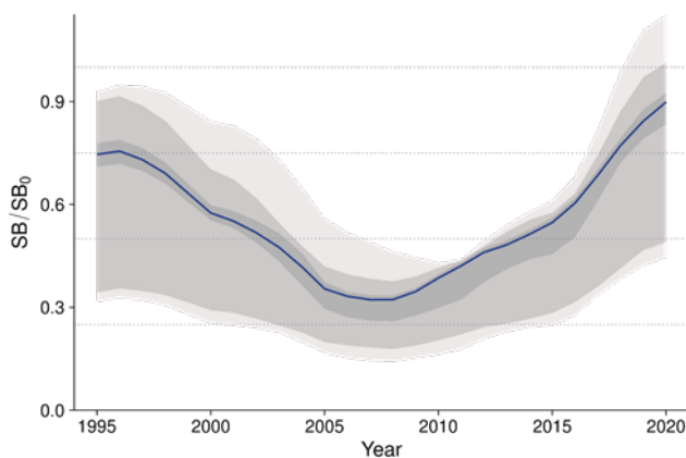
図12. 南太平洋系群の資源評価の中で、SSで推定された南西太平洋におけるヨシキリザメの産卵親魚量の相対値 (1995~2020年) (WCPFC 2022) 縦軸は、未開発時代の産卵親魚量 (SB 0 ) に対する相対値。青線は構造的な不確実性を考慮した全モデルから推定された値の中央値、灰色の影は濃い方から50、80、95%の信頼区間を表す。
