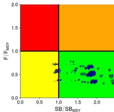
図13. 南太平洋系群の資源評価の中で、SSにより示された神戸プロット (WCPFC 2022) 大きさの異なる丸 (大きいほど重みが大い) は構造的な不確実性を考慮した全モデルから推定された資源状態 (南西太平洋におけるヨシキリザメの相対資源量及び相対漁獲死亡係数の関係) を表す。
