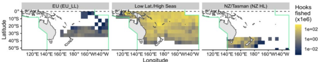
図9. 南太平洋系群の資源評価の中で用いられた空間構造(使用された釣数の空間分布と数)。左図は中緯度域(EUのはえ縄操業エリア)、中図は低緯度域/公海域(日本や台湾船の操業エリア)、右図は高緯度域(ニュージーランドの操業エリア)を表す。
