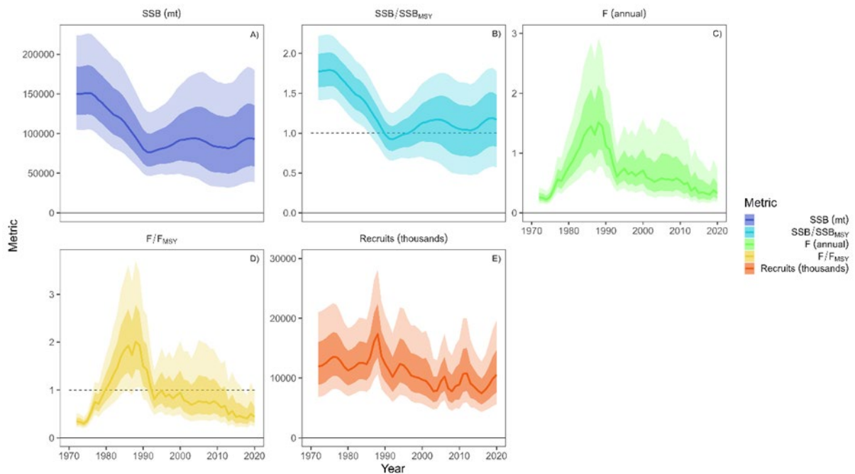
図6. 統合モデル (Stock Synthesis) で推定された北太平洋におけるヨシキリザメの資源状態 (ISC 2022) A) 産卵親魚量 (SSB、トン)、B) 産卵親魚量の最大持続生産量 (MSY) 水準に対する相対値 ( SSB/SSB_{MSY} )、C) 漁獲死亡係数 (F)、D) 漁獲死亡係数の MSY 水準に対する相対値 ( F/F_{MSY} )、E) 加入尾数 (1,000 尾) の年変化 (1971~2020 年)。実線は中央値、濃い影はブートストラッピング手法により推定の不確実性を考慮した場合の 50%、薄い影は 80% の信頼区間、点線は MSY 水準を表す。
