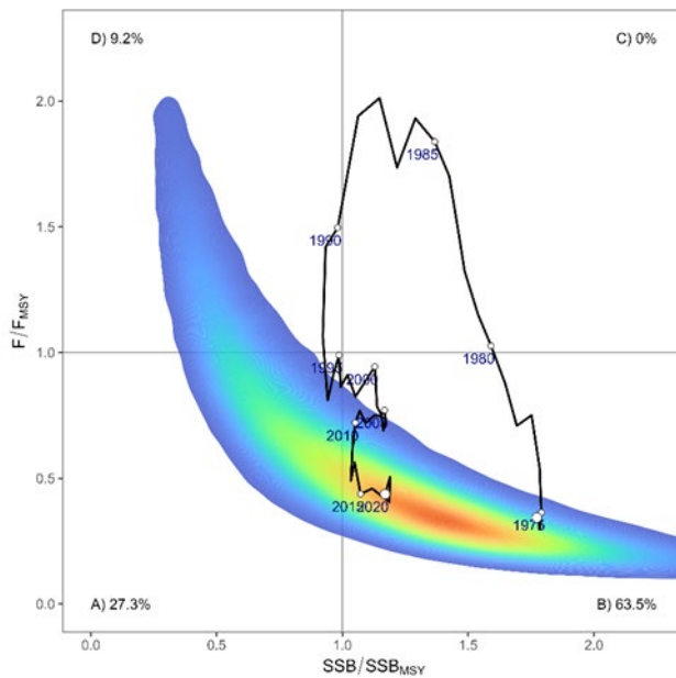
図 7. 北太平洋系群の資源評価の中で、SS により示された神戸プロット (ISC 2022) 白丸及び実線は北太平洋におけるヨシキリザメの相対資源量 (SSB / SSB MSY ) 及び相対漁獲死亡係数 (F / F MSY ) の推移 (1971~2022 年)。 寒暖色は、ブートストラッピング手法により推定の不確実性を考慮した場合の信頼区間を表し、暖色ほどその資源状態にある可能性が高い。
