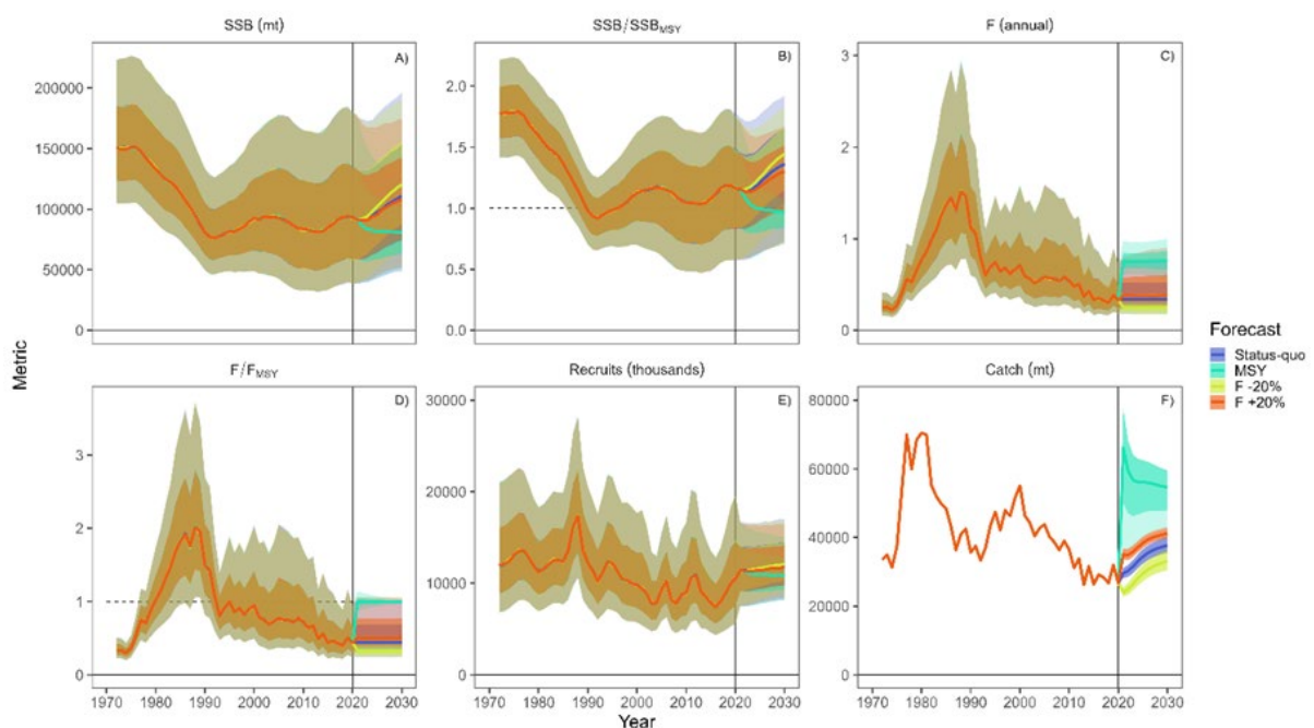
図 8. 北太平洋系群の資源評価の中で、SS により示された将来予測 (ISC 2022) 4 つの異なるシナリオ (①2017~2019 年水準の漁獲死亡係数 (F) : Status-quo、②最大持続生産量の F : MSY、③Status-quo より 20%多い F、④Status-quo より 20%少ない F) で 11 年間 (2020~2030 年) の将来予測を実施。図 A~E の見方については、図 6 を参照。 図 F は漁獲量の年変化 (1971~2020 年) 及び将来予測 (2021~2030 年) を表す。
