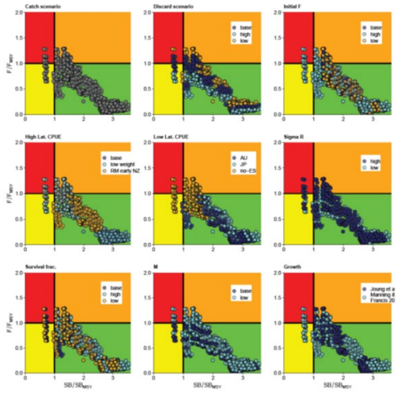
図11. 南太平洋系群の資源評価の中で、SSにより示された神戸プロット (Neubauer et al. 2021) 全グリッド (9種類の異なる不確実性) に対する神戸プロット (漁獲量; 左上図、投棄量; 中央上図、初期の漁獲死亡係数; 右上図、加入量の偏差; 左中図、高緯度域のCPUE; 中央中図、低緯度域のCPUE; 右中図、自然死亡; 左下図、親子関係; 中央下図、成長; 右下図)。異なる色の丸は、異なるシナリオにおける南西太平洋におけるヨシキリザメの相対資源量及び相対漁獲死亡係数の関係。
