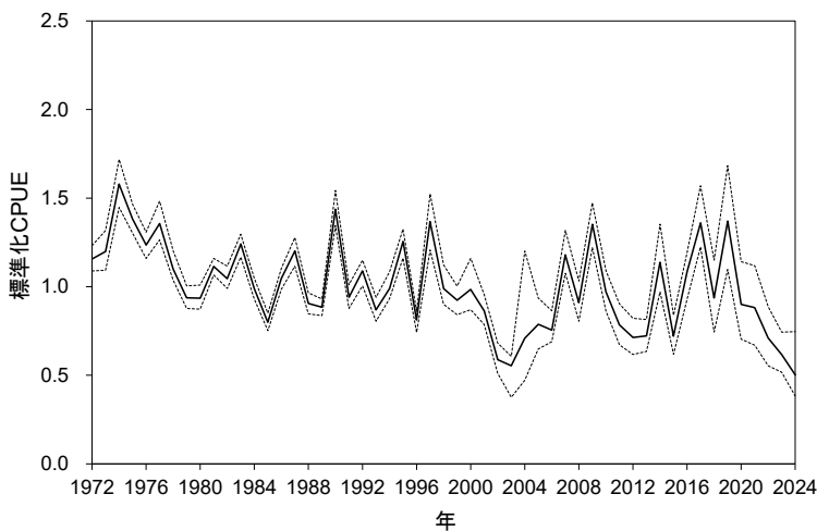
太平洋北区における沖底（かけまわし漁法）の標準化 CPUE（1972～2024 年） 標準化 CPUE は 1 が平均値となるように基準化、 破線はブートストラップ法で推定した 95%信頼区間の上限値と下限値。
