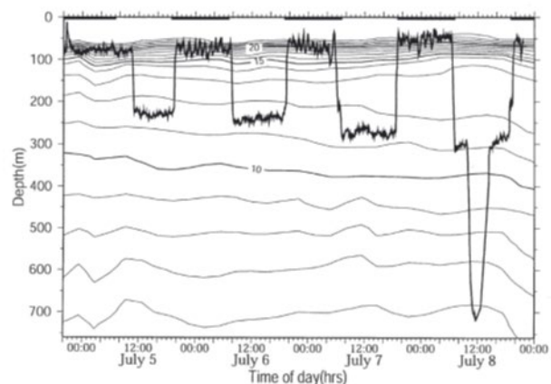
図3. ハチワレの日周鉛直移動（Nakano et al. 2003） 縦軸が遊泳水深、横軸は日にちと時刻を示す。図中の曲線は水温の等深線を示す。
