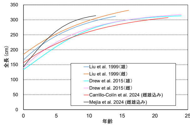
図 4. ニタリの成長曲線 (Liu et al. 1999、Drew et al. 2015、Carrillo-Colín et al. 2024、Mejía et al. 2024 より引用)
